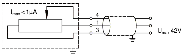
Dargestellte Belegung für ausfahrende Schubstange. Shown configuration for extended position of the actuating rod.
